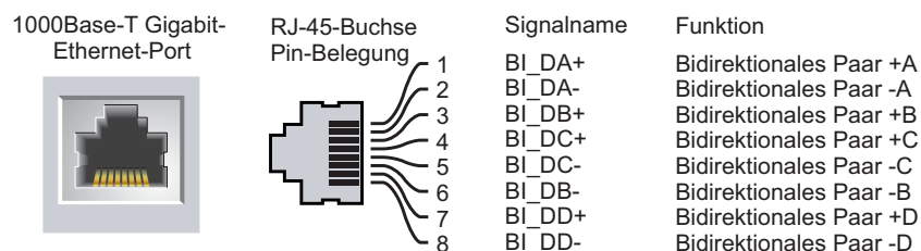
Abbildung 3 Pin-Belegung des Gigabit-Ethernet-Ports
