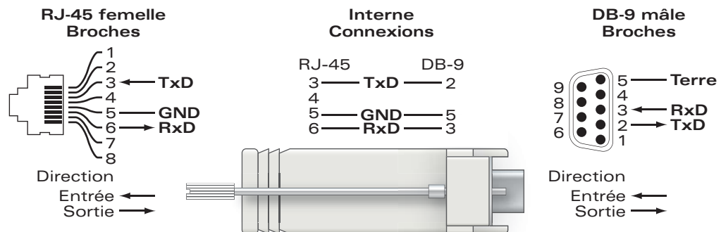
Figure 5 Conversion d'adaptateur modulaire RJ-45 (femelle) vers DB9 (mâle)
